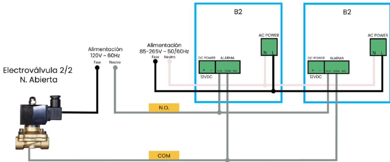
Fig. 6. Conexión típica de dos B2 a electroválvula solenoide
