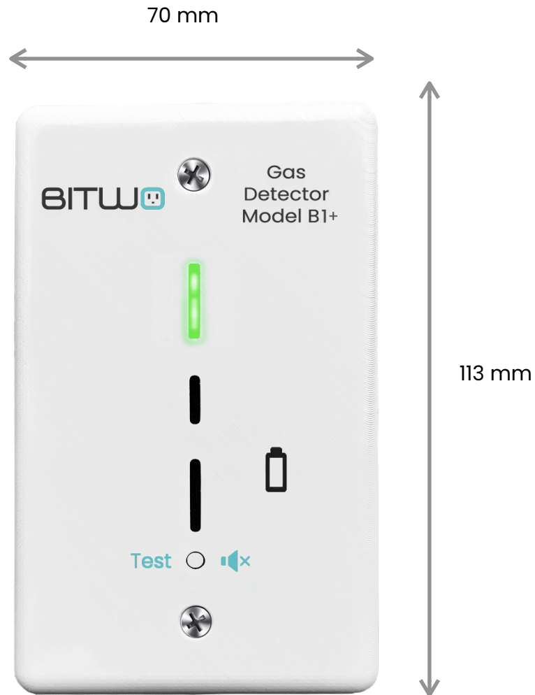
Fig. 3. Medidas del detector
